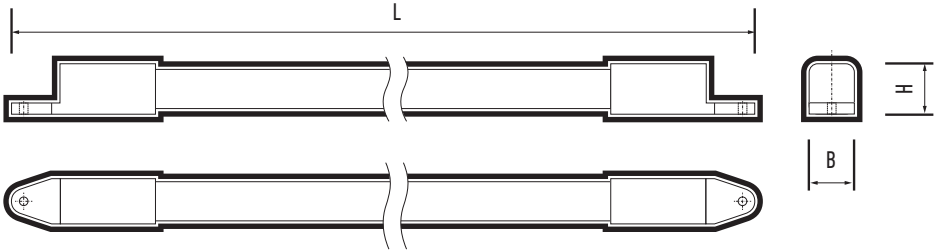
Рис. 1 Светильник PLED T4i
